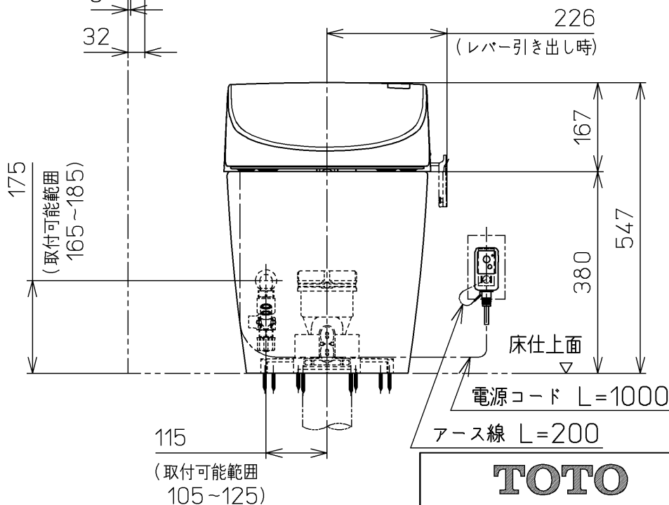
壁給水仕様の場合
